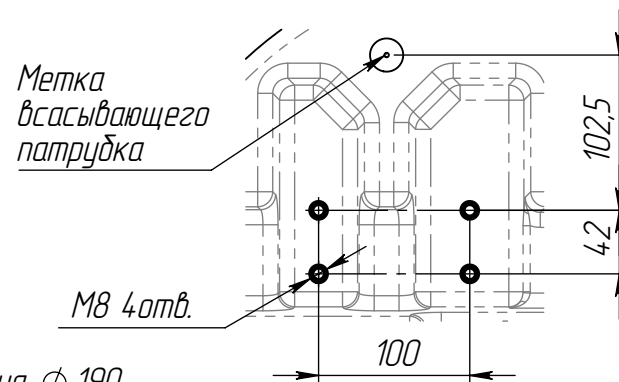
Посадочное место насоса МАСШТАБ 1 : 5
