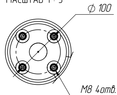
Посадочное место мешалки МАСШТАБ 1 : 5
