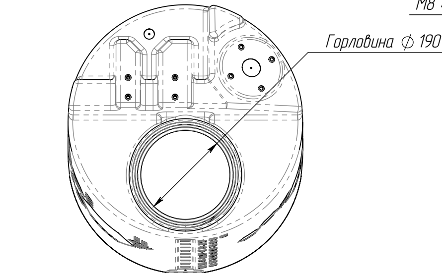
Посадочное место мешалки МАСШТАБ 1 : 5
